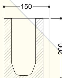
SEZIONE TRASVERSALE
