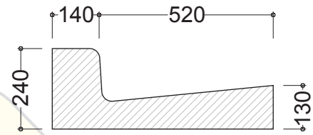
SEZIONE TRASVERSALE
